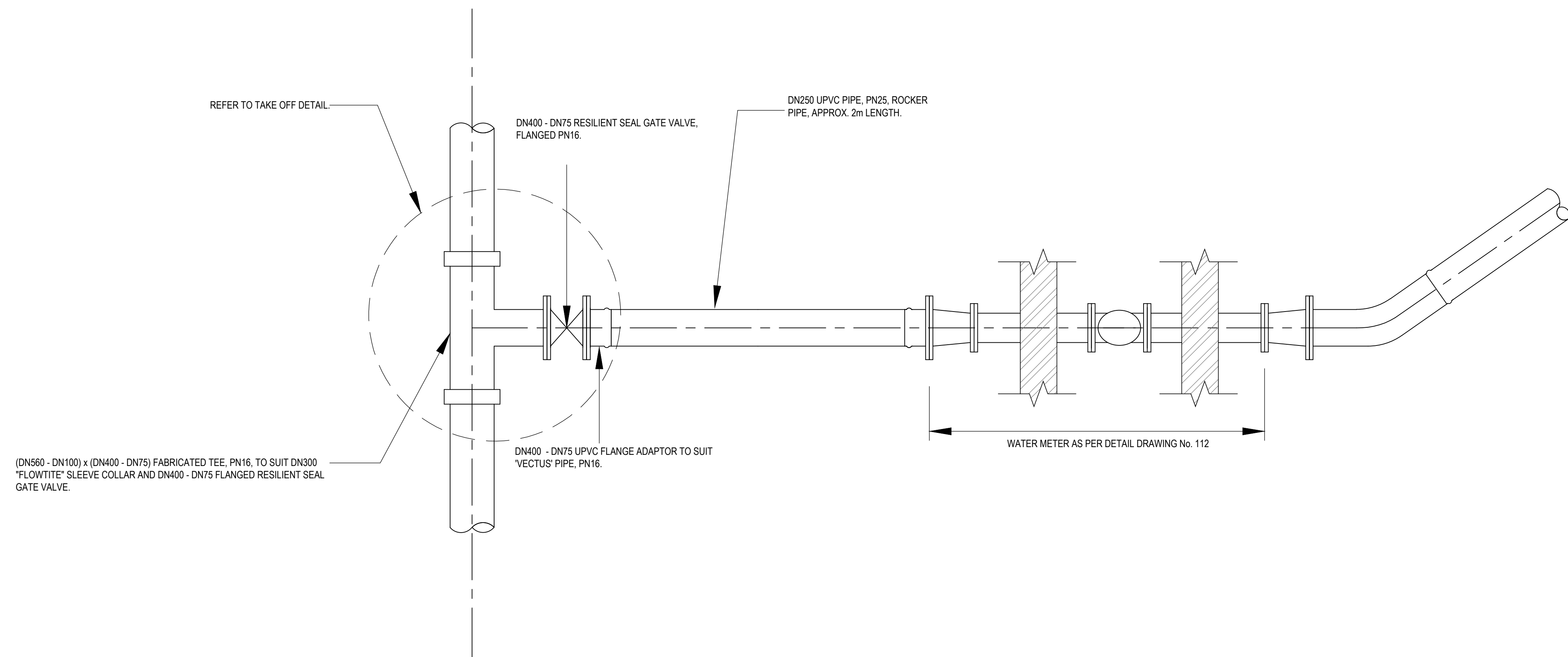
OFF TAKE DETAIL N.T.S.
